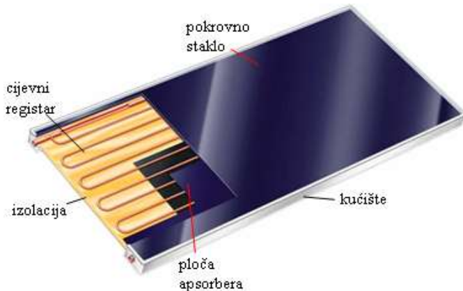
Slika 21. Pločasti kolektor s pokrovnim staklom [9]
